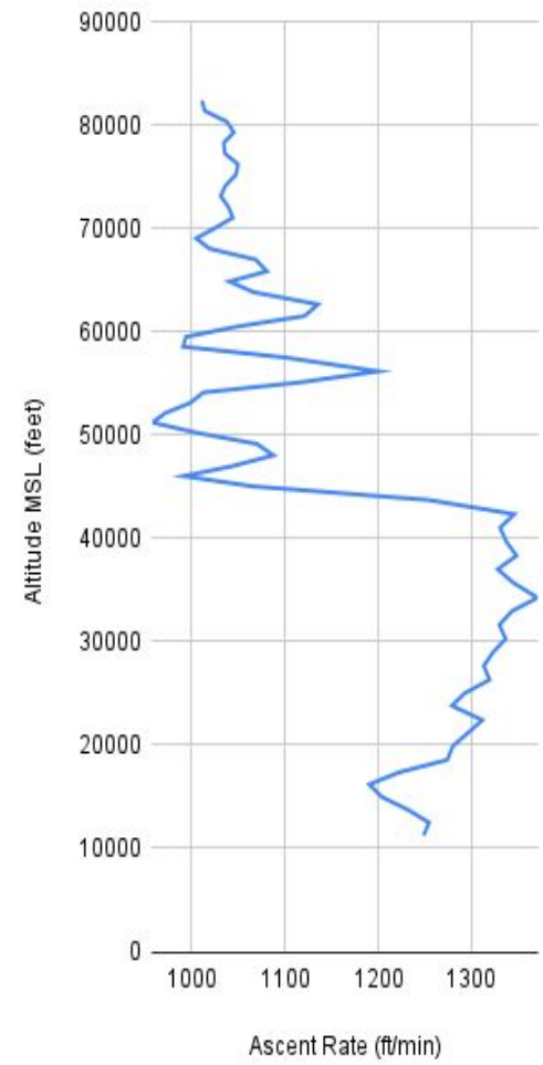
268154_3 Altitude v AscentRate
